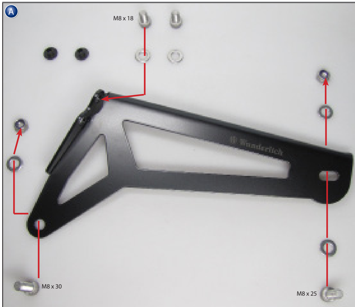
Auspuffhalter BMW R NINE T Bestellnummer 44201-xxx
